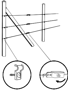
Drahthalter + Drahtspanner
